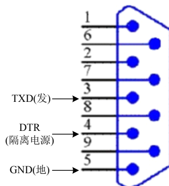
图 5 RS-232 接线示意图
